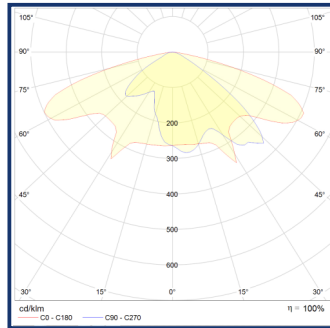
CURVA POLAR
