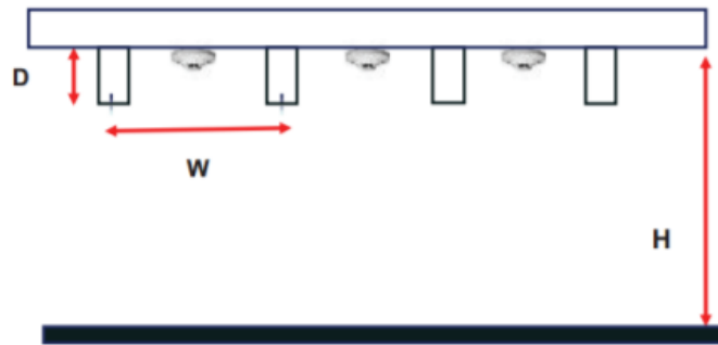
Figura - 3 – Ubicación de sensores en áreas con casetón a la vista opción a
