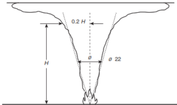
Figura - 5 – Divergencia de columna de humo de un incendio
