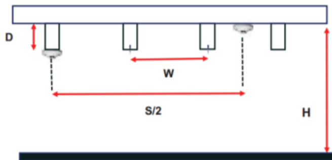
Figura - 4 – Ubicación de sensores en áreas con casetón a la vista opción b
