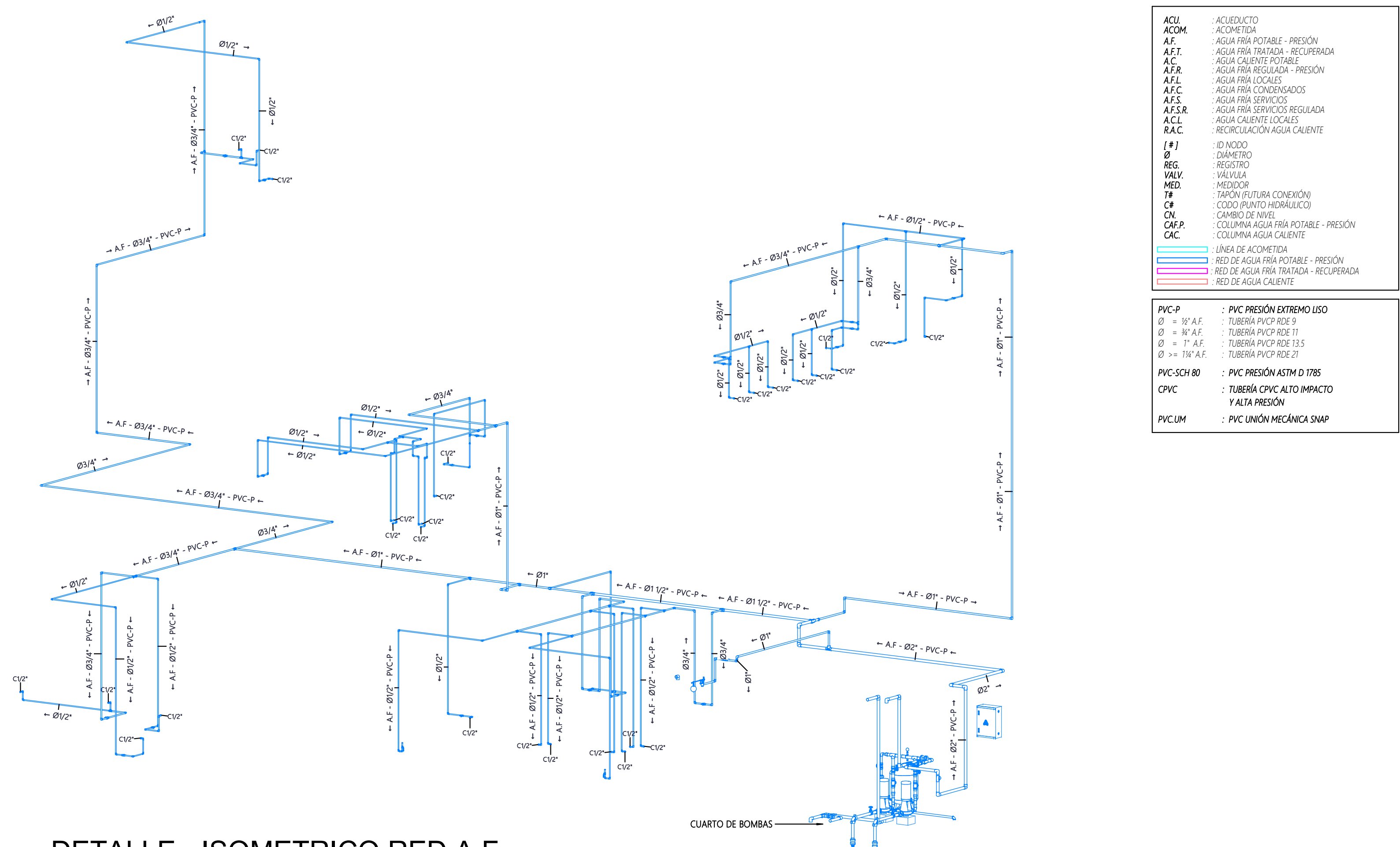
02 DETALLE - ISOMETRICO RED A.F.
