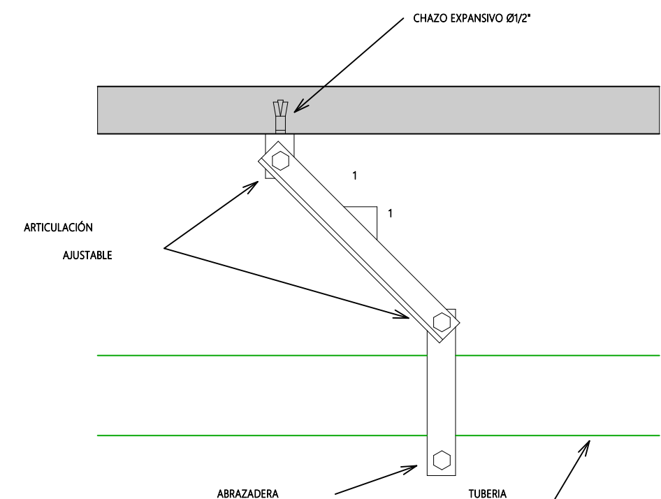
INC - DETALLE - SOPORTE LONGITUDINAL 1 : 10
