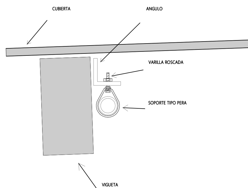
SOPORTE TIPO PERA EN CUBIERTA 1 : 5
