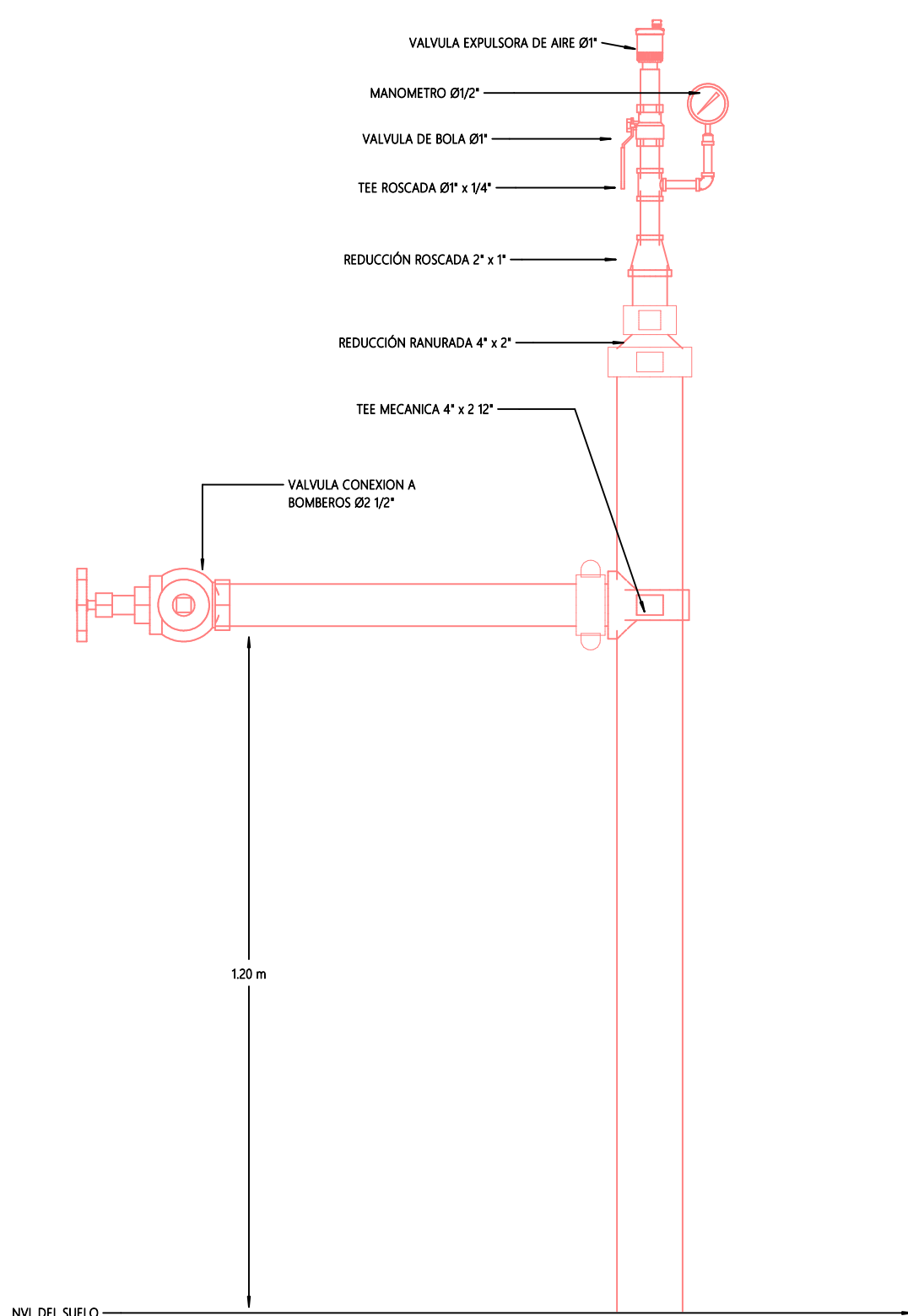
SALIDA 2 1/2" BOMBEROS + VALV. EXPULSORA 1 : 10
