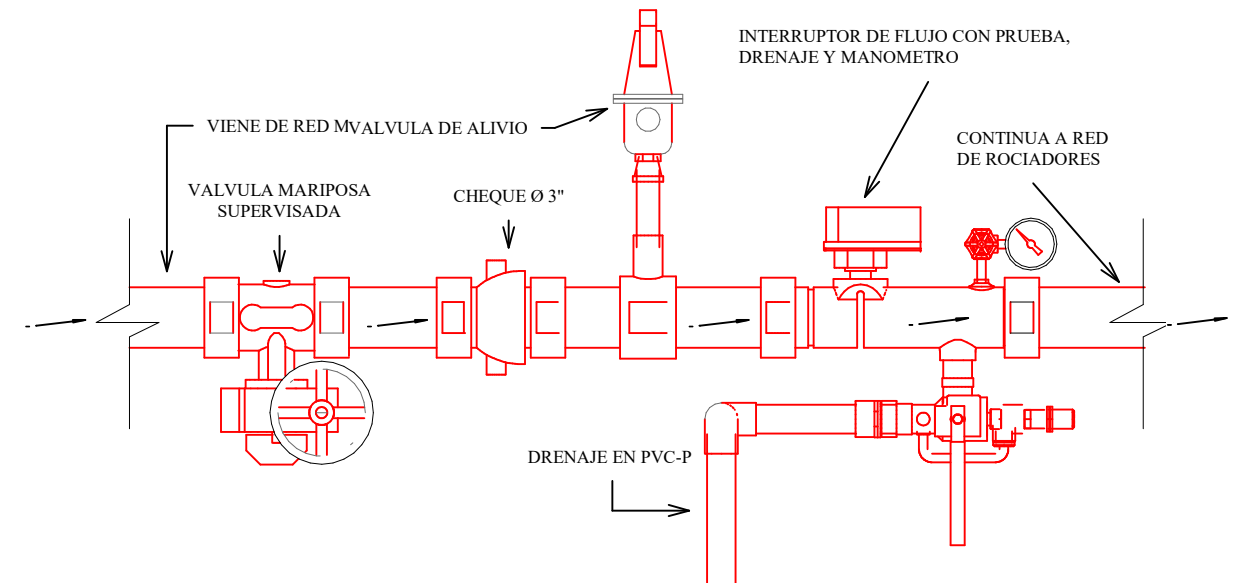
ESTACIÓN DE CONTROL 1 : 20
