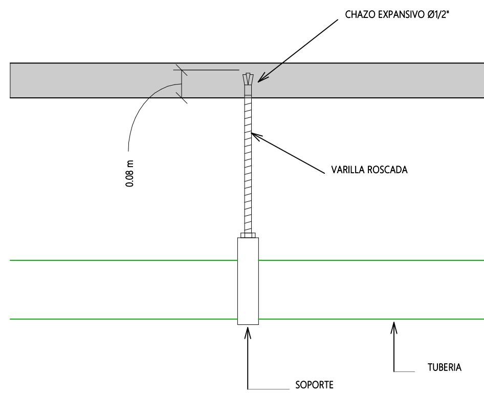
DETALLE - SOPORTERIA TIPO PERA 1 : 10
