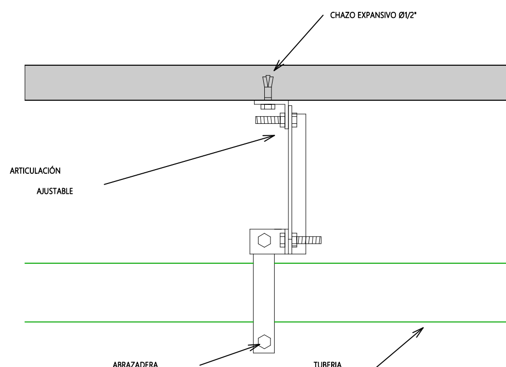
INC - DETALLE - SOPORTE TRANSVERSAL 1 : 10
