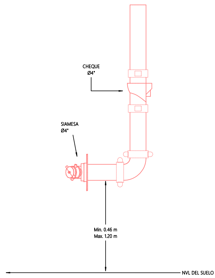
DETALLE SIAMESA Ø4" 1 : 15
